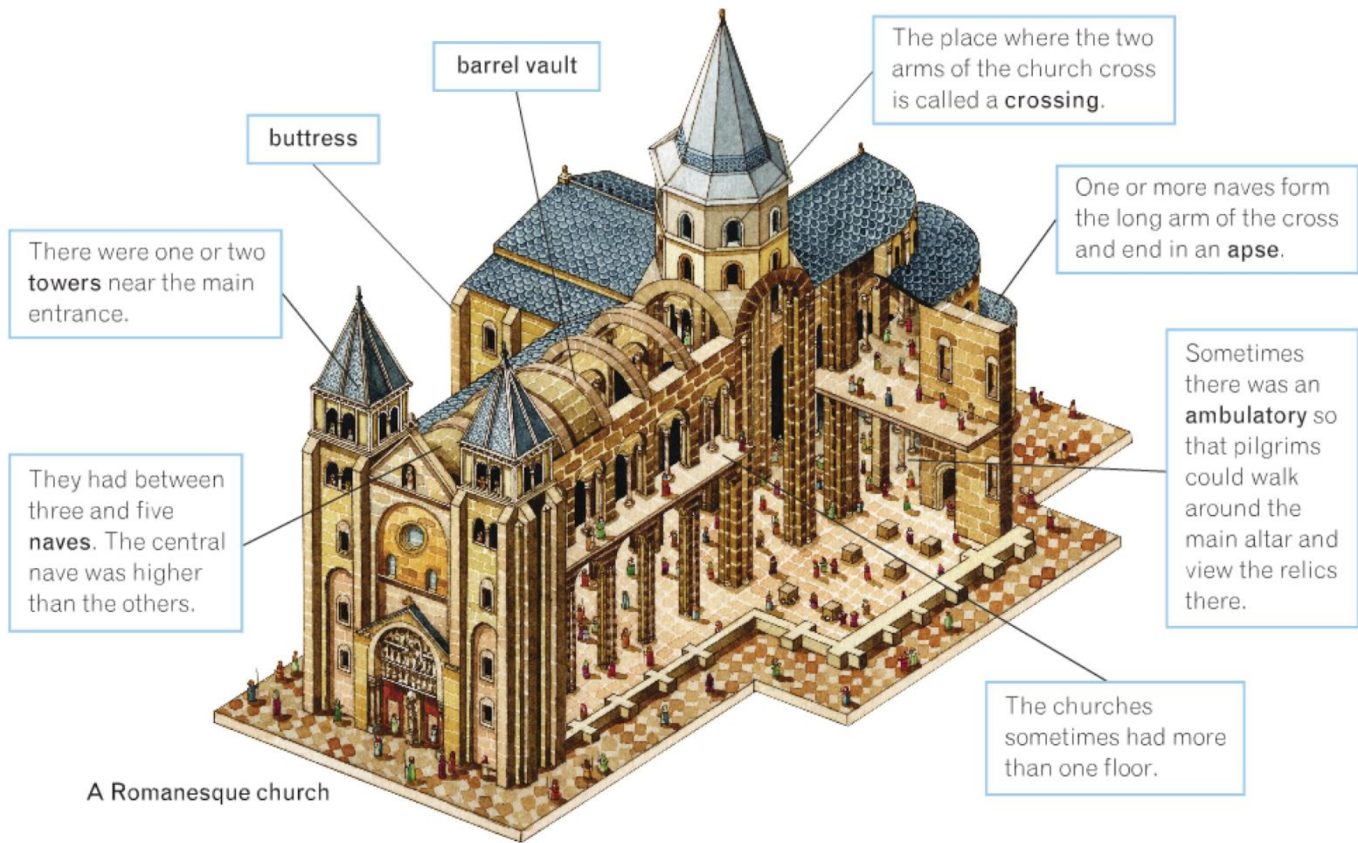
Estrutura arquitetônica de uma igreja Românica.
