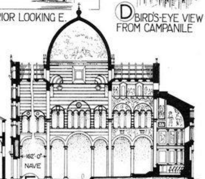
F LONGITUDINAL SECTION
