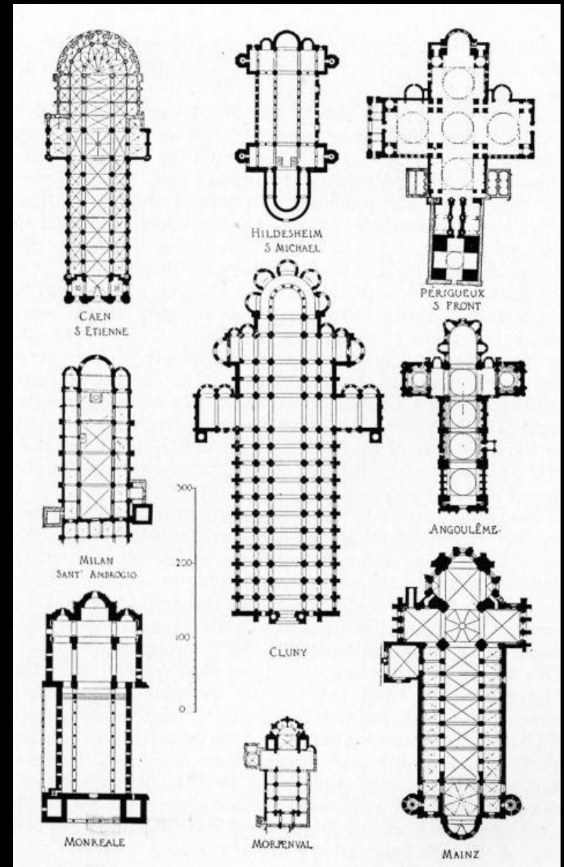
Plantas de Igrejas Românicas
