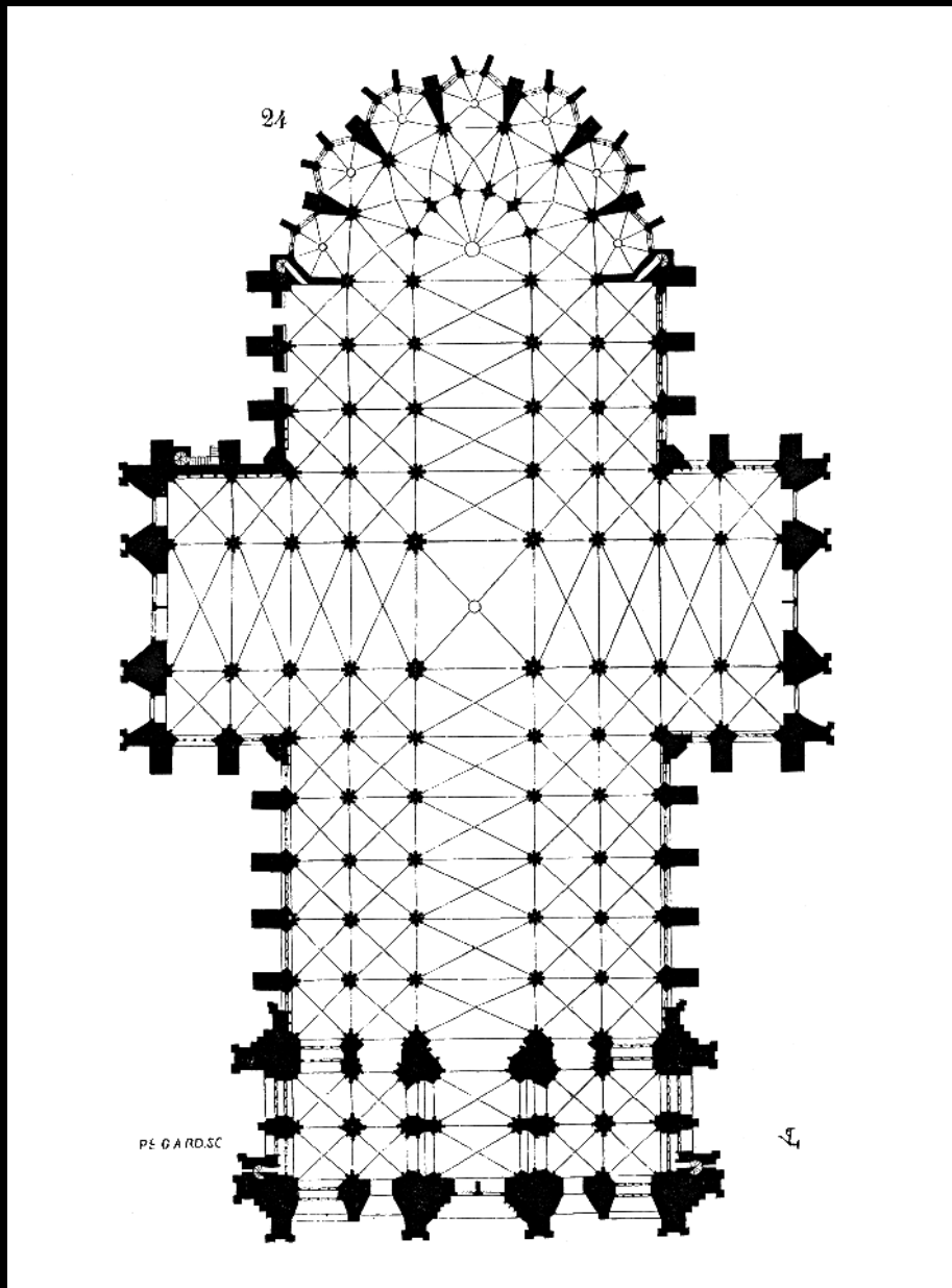
Visão da planta nave central e corte da Igreja de São Pedro em Colônia, Alemanha.
