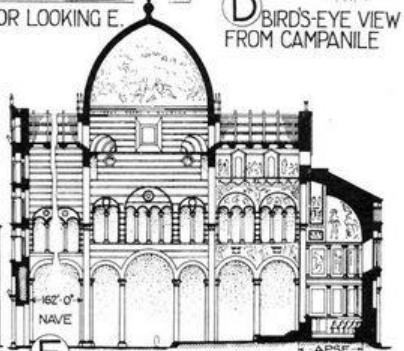
F LONGITUDINAL SECTION
